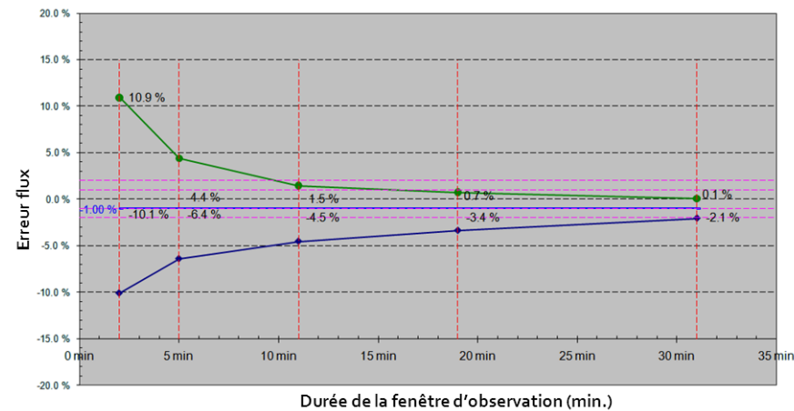
Figure 12.3. Graphique trompette, 24e (dernière) heure d'administration, 1 mL/h
