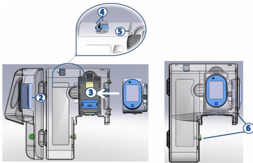
Figure 2.6. Boîtier verrouillable PCA Lock Box 500 : installation
