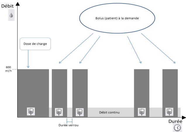
Figure 5.6. Profil de la perfusion PCA
